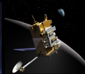
LRO
