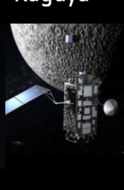
Kaguya
