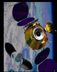
ConeXpress
