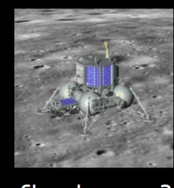
Chandrayaan-2
