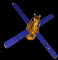
RHESSI
