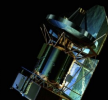
Herschel
