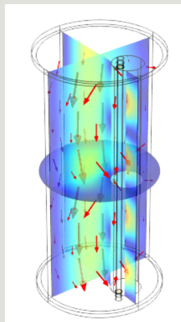
Mode mixing II \nu_c : 1.077 GHz Q_L : 18400 C : 0.14
